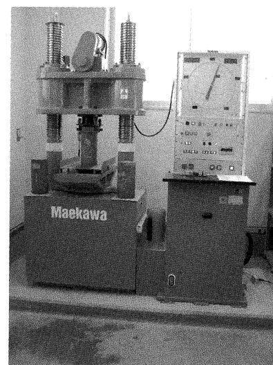
5月に更新した圧縮強度試験機
