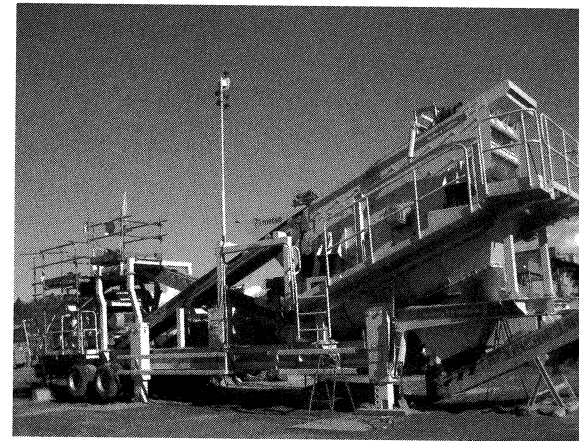
移動式破碎機NW100HP
