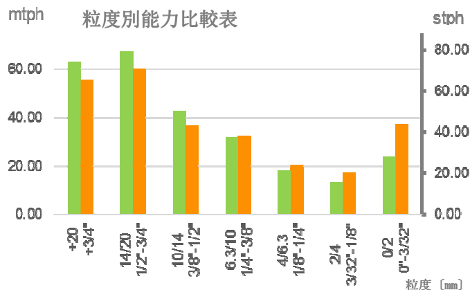
図13 破碎粒度毎の生産量
