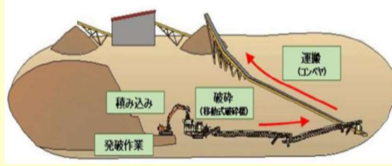
図4 先進工法 (電動式破砕機+フリーライン)
