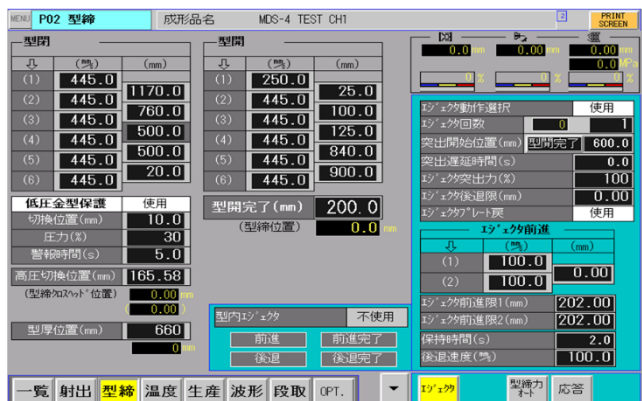
型締画面
