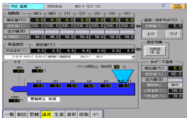
温度画面
